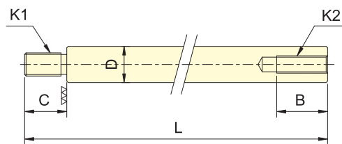
Detail of Draw Bar L = A - G1_{max} - G2_{min} - 4 + C
